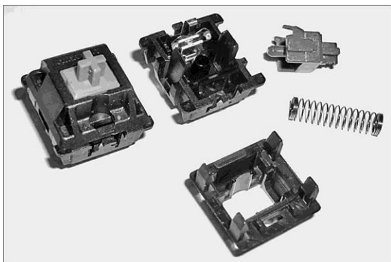
5.3 .сур.Механикалық перне батырмасының механизімі
