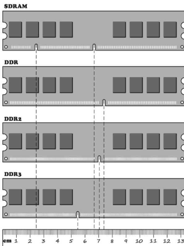
2.8 сур. Ойықтар орналасқан жедел жадының типтері
