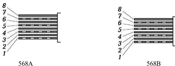
Рис. 11.3. Два стандарта: EIA/TIA-568A и EIA/TIA-568B
