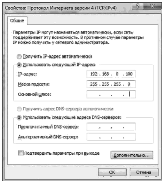
11.11.сур.Қасиеттер Сұхбат терезесі:4 нұсқаның Интернет хаттамасы
