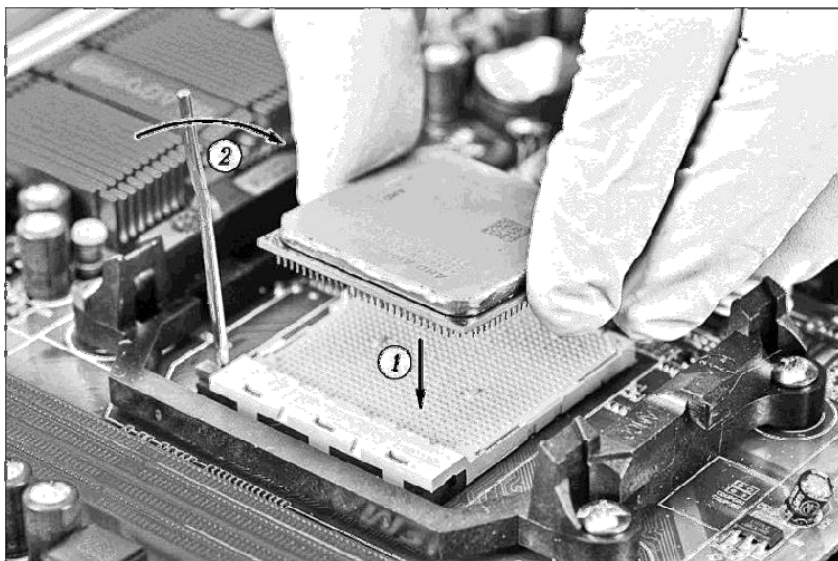
2.5 .сур. Орталық процессорды орнату
