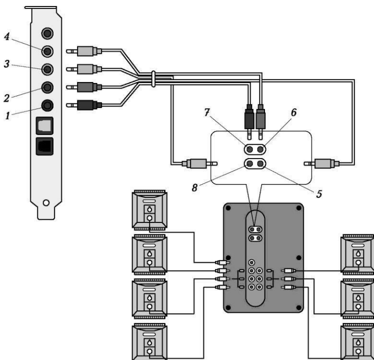
4.2. сур. Картаның стерео шығыстары – 7.1 жүйесі бойынша барлық төрт шығыс арқылы қосу (7 ...8 – арналар)
