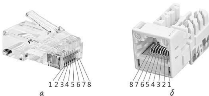
11.2 .сур. Коннектор және RJ45 ағытпа
