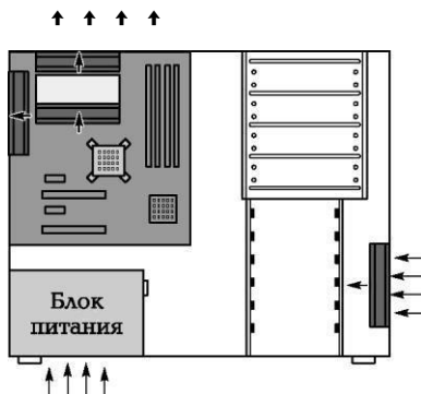
7.1. сур. Корпустың ішіндегі фронталды желдеткіш
