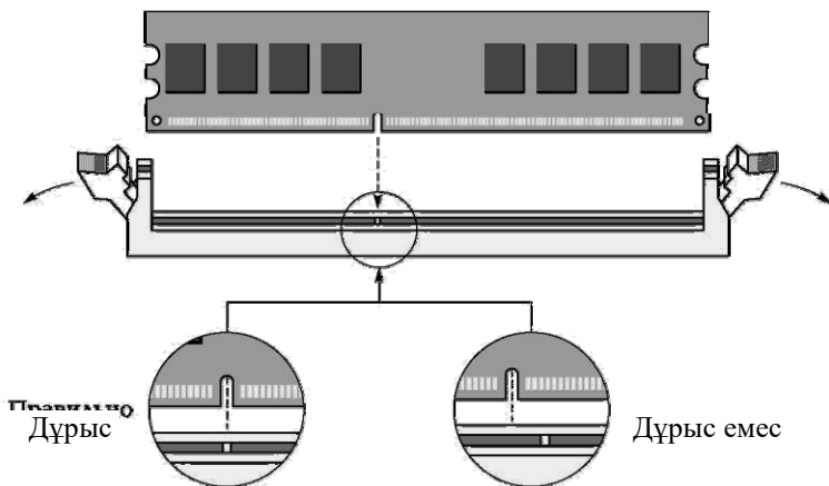
2.9 сур. Слоттағы кілт және жедел жадыдағы ойық
