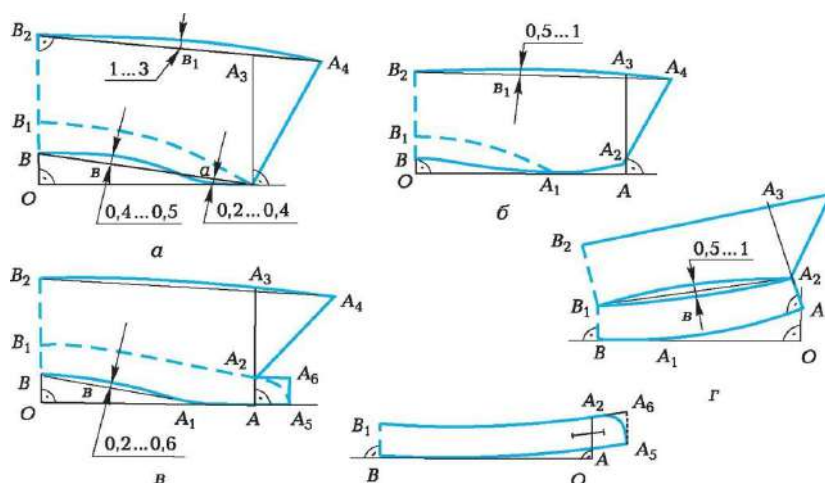
8.10 -сур. Ер балаларға арналған киім жағасының құрылымының сызбаларын құрастыру
