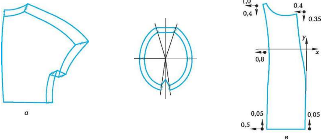
15.1 сурет. Сызбаүлгілер градациясы
