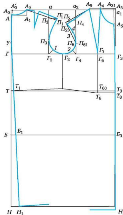
7.7. суреті. Қыз балаға арналған қондырма жеңі бар иықты бұйымның негіз сызбасы
