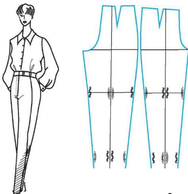
12.29 сурет. Балтырдан жоғары және төмен шалбарлардың артқы жартыларындағы көлденең және көлбеу кептеулер. Ақау көбінесе тар шалбарларда кездеседі
