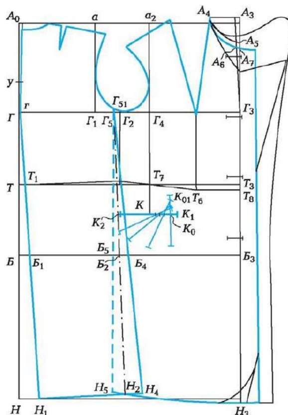
5.14. Бұйымдардағы бүйірлік сызықтарды артқы қиылған жағымен ресімдеу. Борттық сызық пен қалта сызығын безендіру
